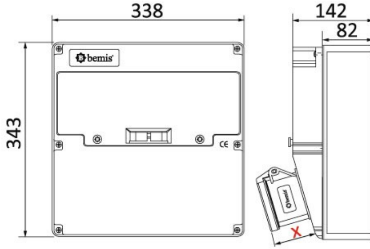
(X) Ölçüleri / Dimensions (mm)
