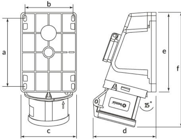
Ölçüler / Dimensions (mm)
