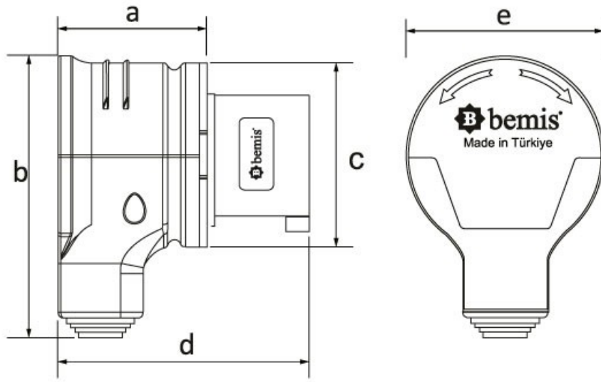
Ölçüler / Dimensions (mm)
